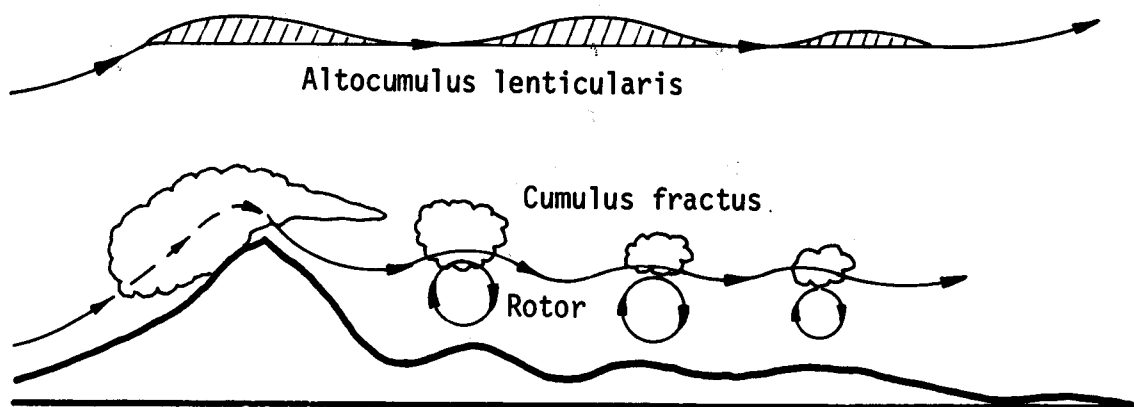
Figur 9 - Wellen- und Rotorenbildung
