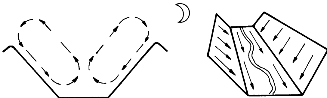
Figur 2 - Bergwind
