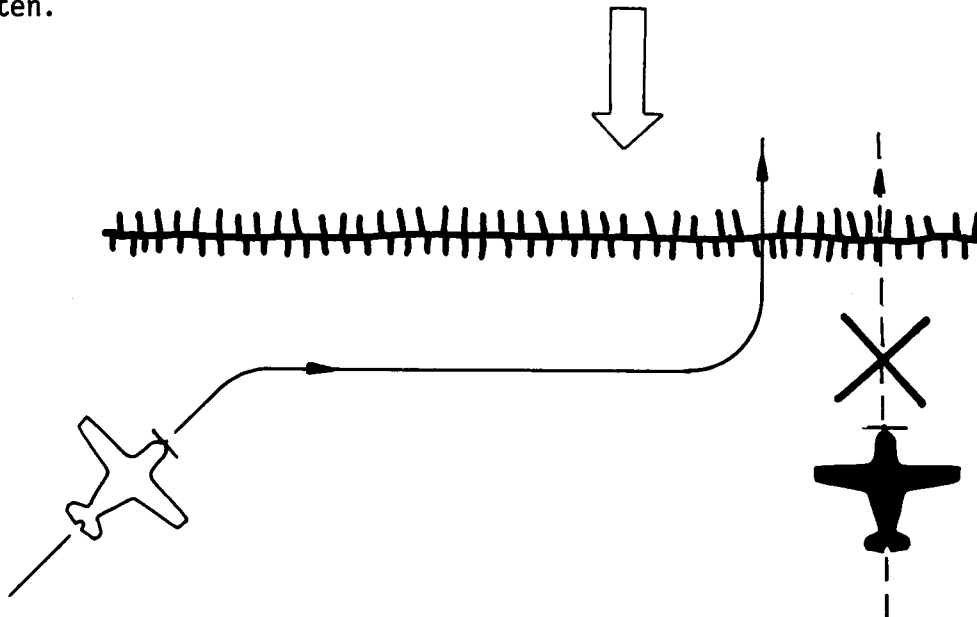
Figur 26 - Ueberfliegen eines Bergkammes (von oben gesehen)
