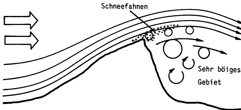
Figur 6 - Auswirkung der Turbulenz bei sehr starkem Wind
